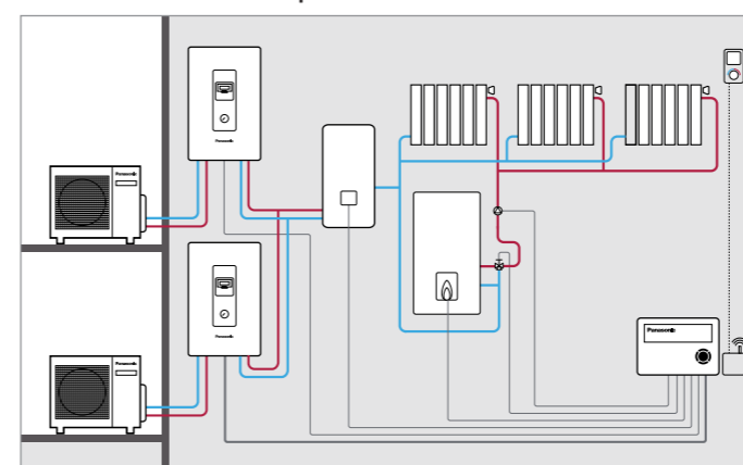
2 тепловых насоса + бойлер с PAW-HPM12ZONE-U
