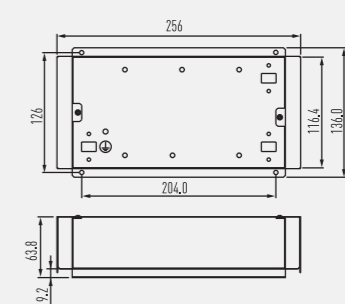
КОНТРОЛЛЕР ВВОДА / ВЫВОДА SERI-PARA I / O ДЛЯ КАЖДОГО ВНУТРЕННЕГО БЛОКА (CZ-CAPBC2)
