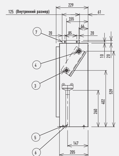
Габаритные размеры: мм
