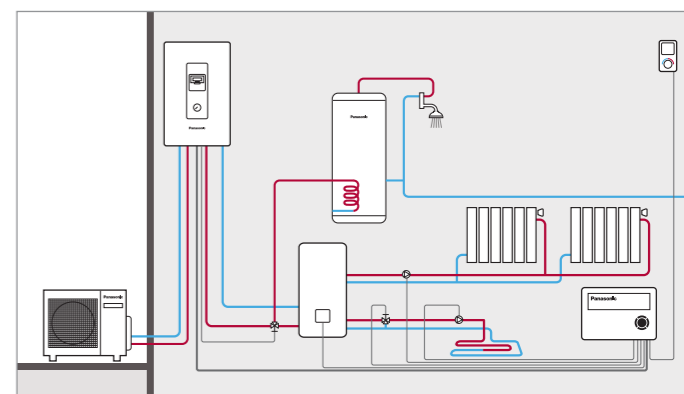
Управление температурой в 2 зонах + ECS с PAW-HPM12ZONE-U
