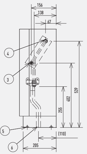
Габаритные размеры: мм
