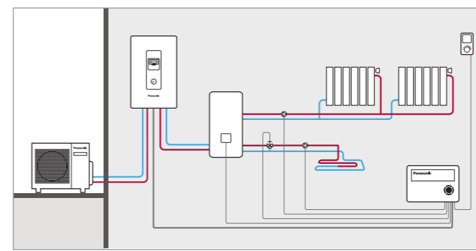
Управление температурой в 2 зонах с PAW-HPM12ZONE-U
