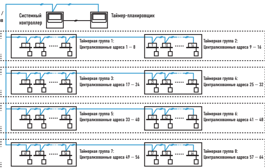
Пример подключения 2 (питание от центрального контроллера)
