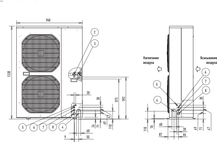
ВИД СПЕРЕДИ
