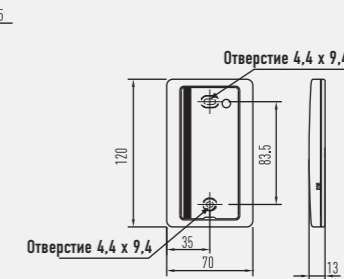
Отдельный приемник для пульта ДУ
