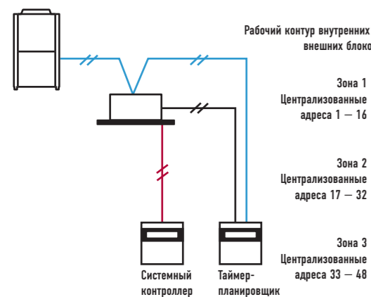
Пример подключения 1 (питание от внутреннего блока)
